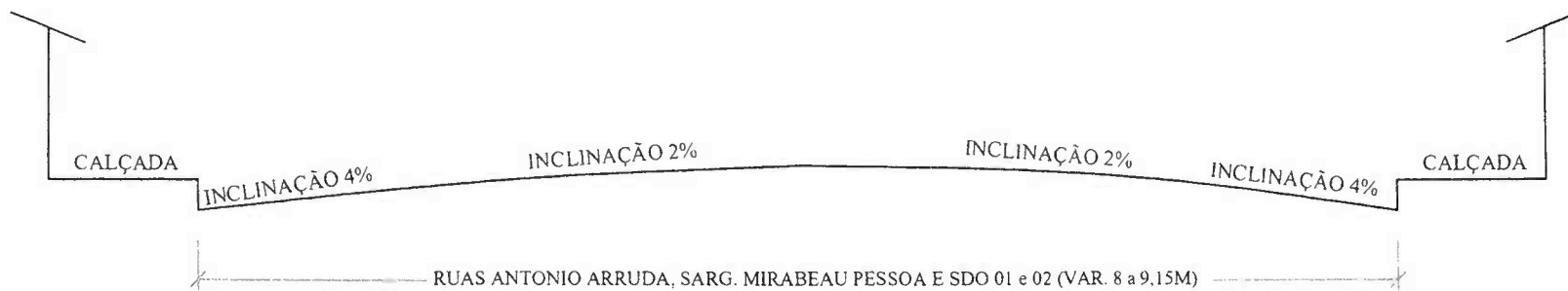
2 SEÇÕES TRANSVERSAIS DAS RUAS ESCALA: 1:50
