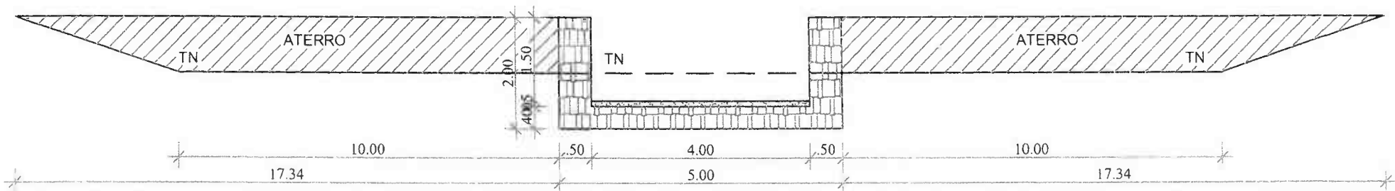
1 SEÇÃO TRANSVERSAL PADRÃO DO CANAL ESCALA: 1:100
