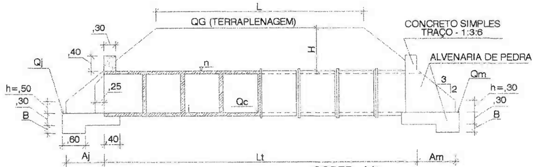
CORTE - AA' ESC.: S/ESC
