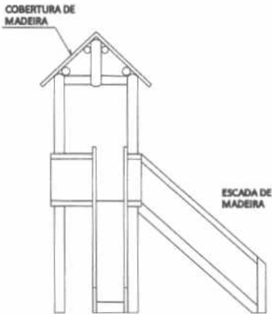
02 VISTA 4 ESCALA — 1 : 100
