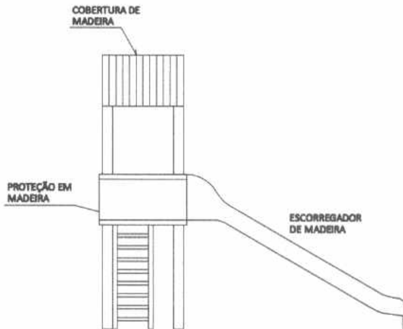
02 VISTA 1 ESCALA — 1 : 100
