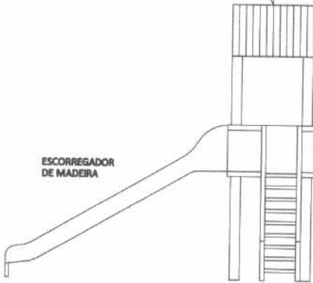
01 VISTA 2 ESCALA — 1 : 100
