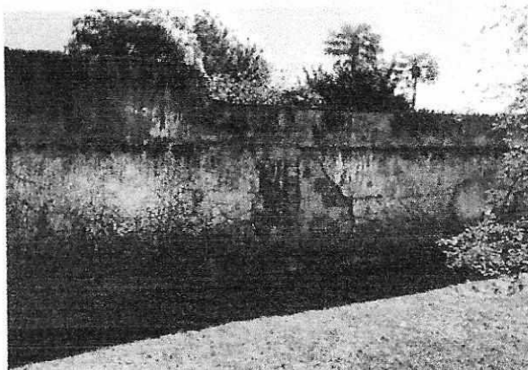
Foto 05: Muro com deslocamento do revestimento argamassado
