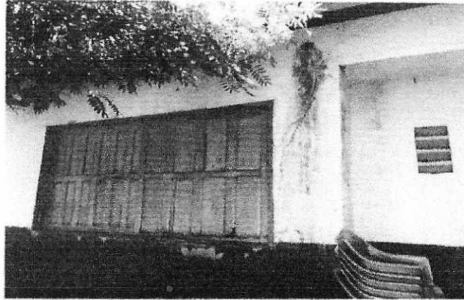
Foto 06: Trincas na alvenaria da edificação.
